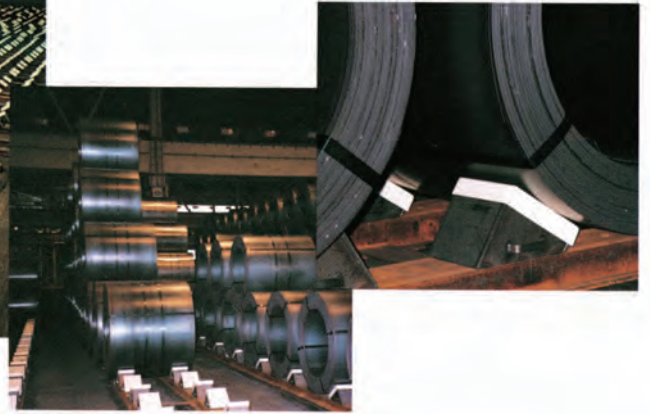
■ ピッチ可変式コイルスキット&三角ストッパー
